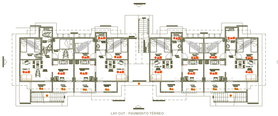
Figura 10: Layout do Empreendimento Res. Liberdade I – Pavimento Térreo.
