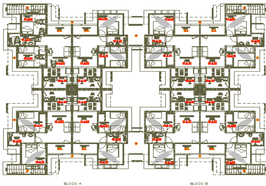
Figura 14: Layout do Empreendimento Res. Liberdade III – Segundo Pavimento.
