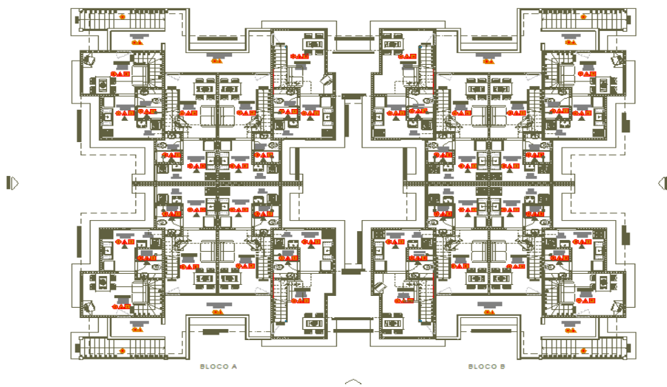
Figura 13: Layout do Empreendimento Res. Liberdade III – Primeiro Pavimento.
